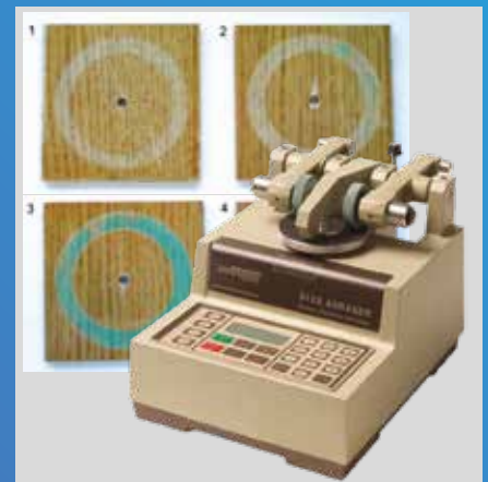
Taber Test: Ermittlung der Abriebbeständigkeit nach verschiedenen Normen
